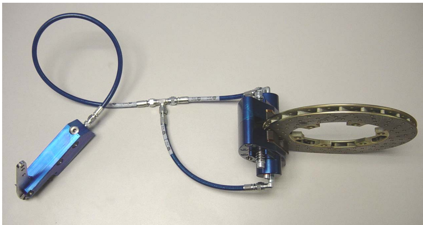
PHOTO VUE DE DESSUS DU SYSTÈME COMPLET PHOTO FROM ABOVE OF COMPLETE SYSTEM
